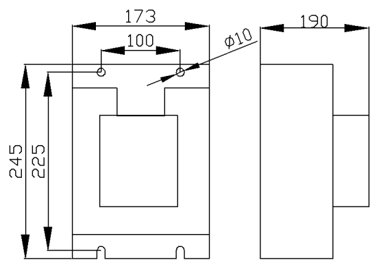
图A（B160散热器）
