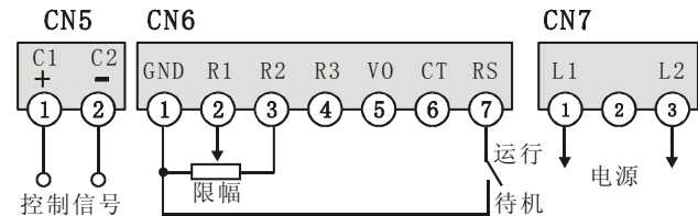
图4：带限幅功能的自动控制接线图
