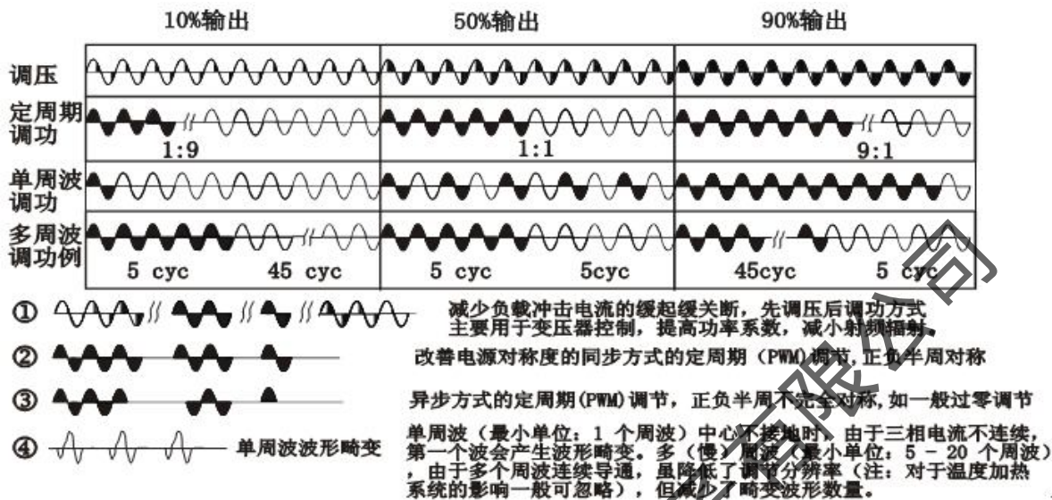
图 11 调压 调功的负载电压电流波形对比
