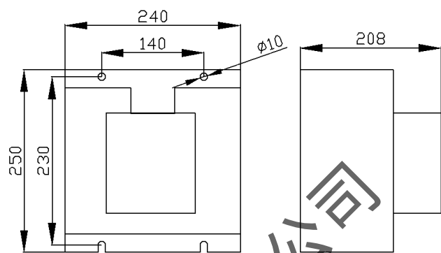
图B（B227散热器）
