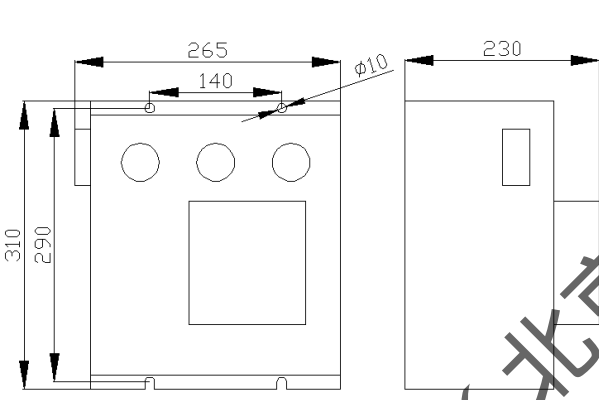
图C（B301散热器）
