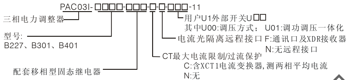
图 1: PAC03I 系列型号定义
